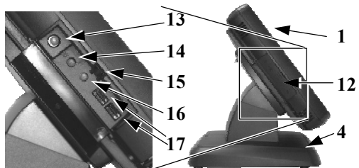
Inside touch open door
